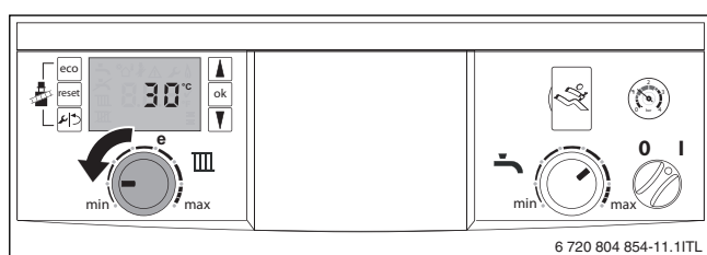
Fig. 12 Fremløbstermostat på 30 °C
