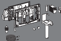
Geberit DuoFresh modul med automatisk aktivering af lugtudsugning og indsats til Geberit DuoFresh sticks
